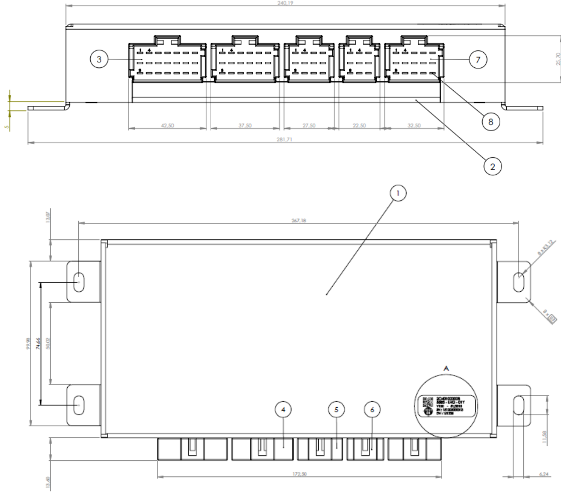
Şekil 19: oMux 22x24 montaj için ölçüler
