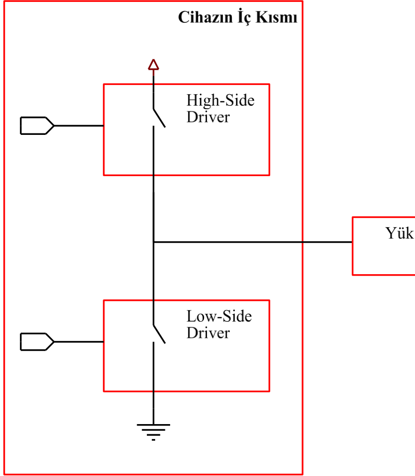
Şekil 15: Tipik “Half-Bridge” Çıkış Montaj bağlantısı
