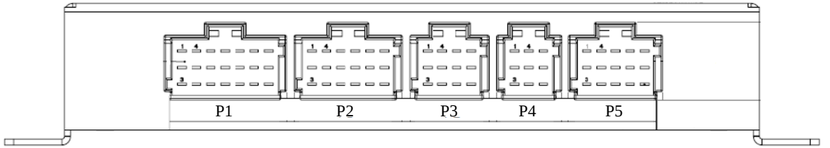
Şekil 9: Konnektörlerin görünümü
