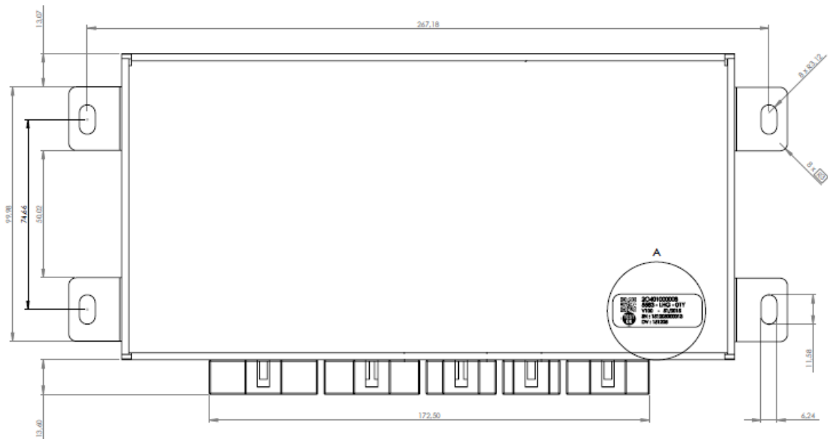
Şekil 17: 22x24 oMux teknik çizim görseli
