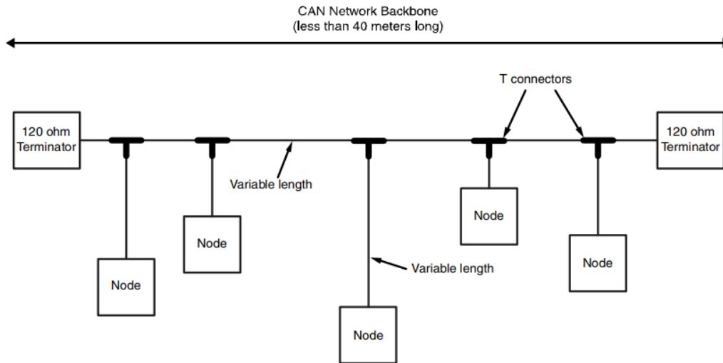
Şekil 16: CAN bağlantısı
