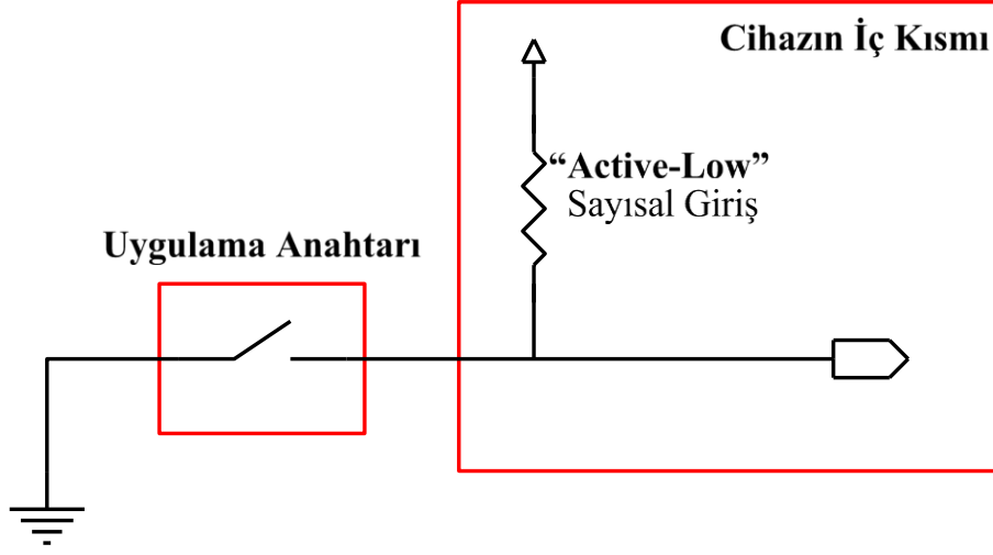
Şekil 11: Aktif-Low Sayısal Giriş
