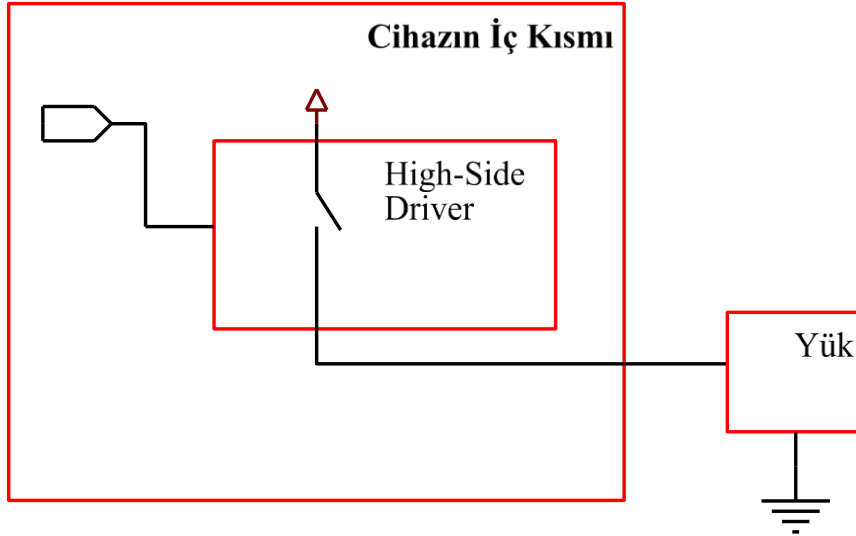
Şekil 14: Tipik “High-Side” Çıkış Montaj bağlantısı
