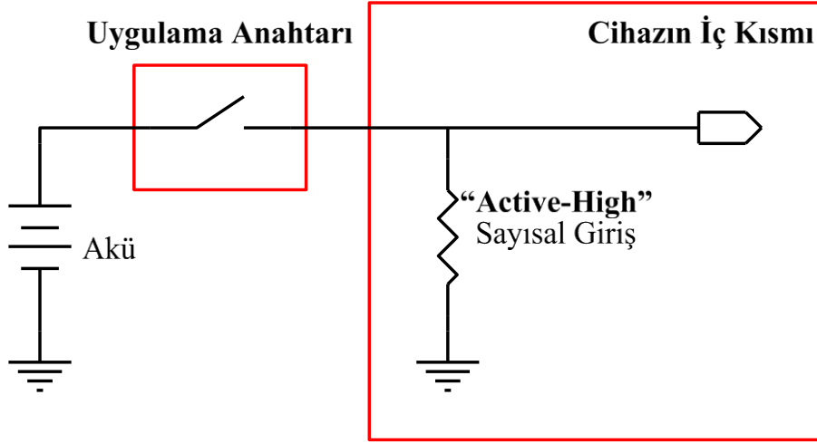
Şekil 10: Aktif-High Sayısal Giriş
